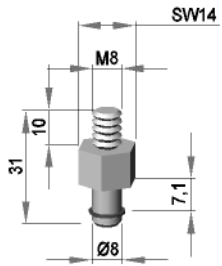
Rollenaufnahme RA 8 / 15 / M8
