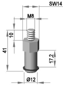
Rollenaufnahme RA 12 / 20 - 30 / M8
