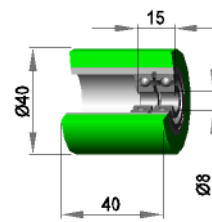
Silikon 90 shore
