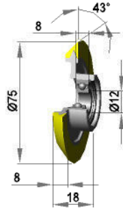
Silikon 70 shore
