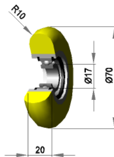
Silikon 70 shore
