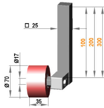
Rollenhalterung □ 25 drehbar mit Rolle R 17 / 35 / 70 / PO
