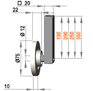
drehbare Führungsrollenhalterung mit Rolle F 12 / 10 / 75 / PO
