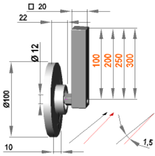
Führungsrollenhalterung □ 20 mit Rolle F 12 / 10 / 100 / AL
