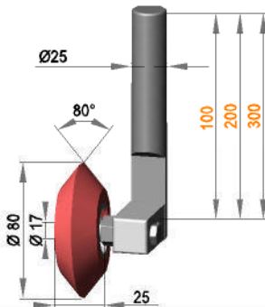
Rollenhalterung Ø25 drehbar mit Rolle ER 17 / 25 / 80 / PO
