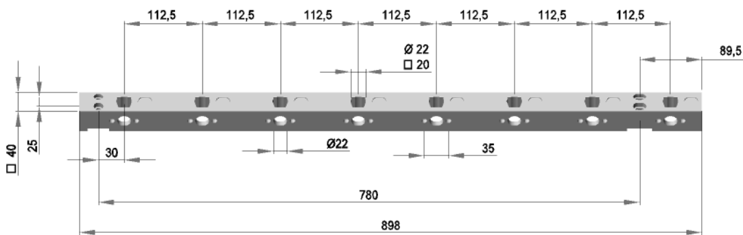
Werkzeugträger für Höhenverstellung
