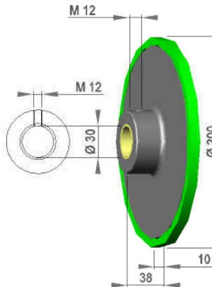
Silikon 90 shore
