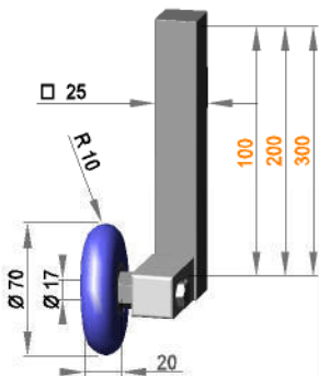
Rollenhalterung □ 25 drehbar mit Rolle RR17 / 20 / R10 / AL
