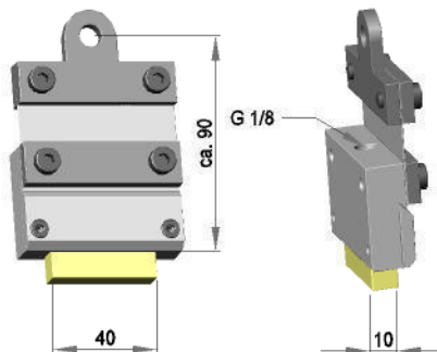
gefederter Filzhalter, Montage oben, Filz 100 mm FH / G / 100
