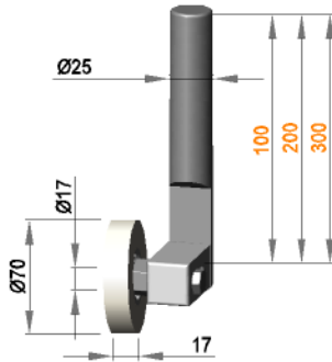
Rollenhalterung Ø25 drehbar mit Rolle R 17 / 25 / 70 / S50R
