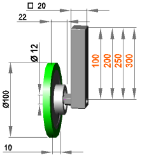
drehbare Führungsrollenhalterung mit Rolle F 12 / 10 / 100 / S90Gr
