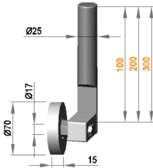
Rollenhalterung Ø25 drehbar mit Rolle R 17 / 25 / 70 / S30B
