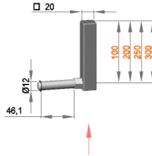
Ansicht Pfeilrichtung
