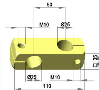
Kreuzklemmstück - links KRR 25 /L / MS
