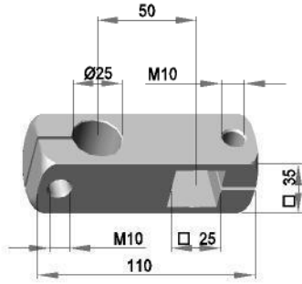
Kreuzklemmstück - rechts
