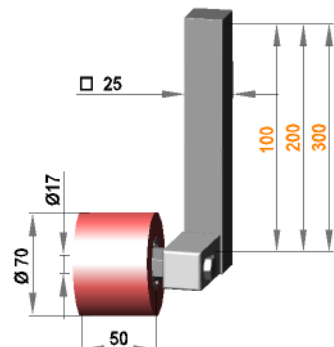
Rollenhalterung □ 25 drehbar mit Rolle R 17 / 50 / 70 / PO
