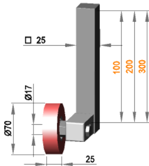
Rollenhalterung □ 25 drehbar mit Rolle R 17 / 25 / 70 / PO
