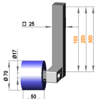
Rollenhalterung □ 25 drehbar mit Rolle R 17 / 50 / 70 / AL
