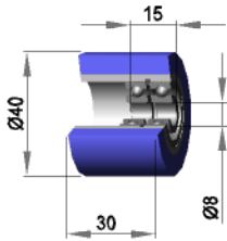
Silikon 30 shore
