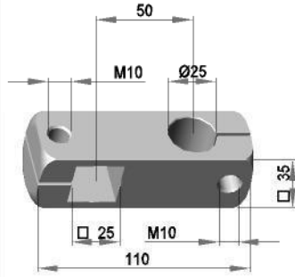
Kreuzklemmstück - links
