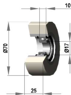
Polyamid
