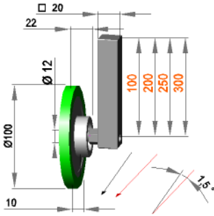
Führungsrollenhalterung 1,5° R mit Rolle F 12 / 10 / 100 / S90Gr
