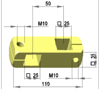
Kreuzklemmstück - links
