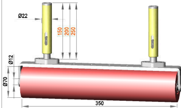
Gefederte Rollenhalterung mit Rolle R 12 / 350 / 70 / S90Gr
