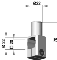
Einfachklemmstück EKU 70
