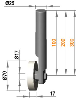
Rollenhalterung Ø25 mit Rolle R 17 / 25 / 70 / S50R
