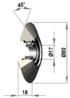
Polyamid
