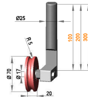
Rollenhalterung Ø25 drehbar mit Rolle NR17 / 20 / R5 / PO
