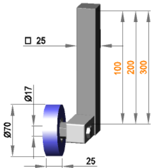
Rollenhalterung □ 25 drehbar mit Rolle R 17 / 25 / 70 / AL
