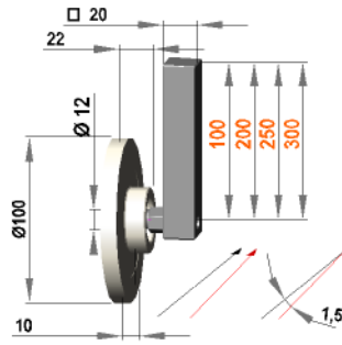
Führungsrollenhalterung □ 20 mit Rolle F 12 / 10 / 100 / PO
