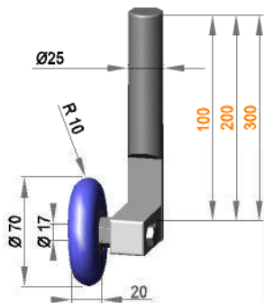
Rollenhalterung Ø25 drehbar mit Rolle RR17 / 20 / R10 / AL
