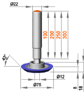
Feststehende Rollenhalterung mit Rolle ERL 12 / 16 / R43 / S30B
