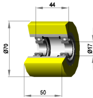
Silikon 70 shore
