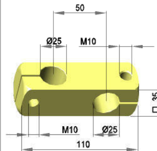
Kreuzklemmstück - rechts KRR 25 /R / MS
