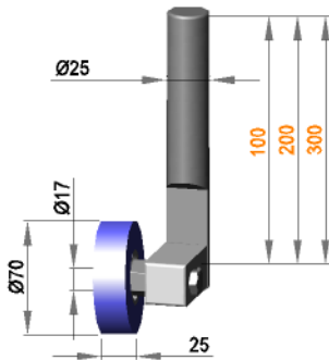
Rollenhalterung Ø25 drehbar mit Rolle R 17 / 25 / 70 / AL
