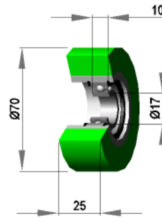
Silikon 90 shore
