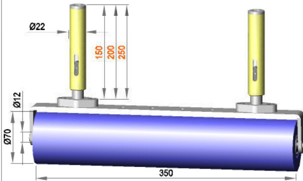
Gefederte Rollenhalterung mit Rolle R 12 / 350 / 70 / S70G
