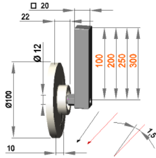
Führungsrollenhalterung 1,5° R mit Rolle F 12 / 10 / 100 / PO
