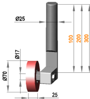
Rollenhalterung Ø25 drehbar mit Rolle R 17 / 25 / 70 / PO
