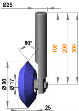
Rollenhalterung Ø25 mit Rolle ER 17 / 25 / 80 / AL
