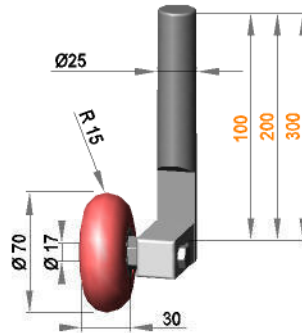
Rollenhalterung Ø25 drehbar mit Rolle RR17 / 30 / R15 / PO
