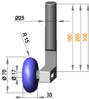
Rollenhalterung Ø25 drehbar mit Rolle RR17 / 30 / R15 / AL
