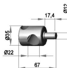
Klemmstück KR 22
