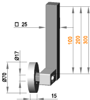
Rollenhalterung □ 25 drehbar mit Rolle R 17 / 25 / 70 / S30B
