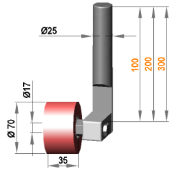
Rollenhalterung Ø25 drehbar mit Rolle R 17 / 35 / 70 / PO
