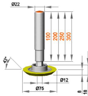
Feststehende Rollenhalterung mit Rolle ERL 12 / 16 / R43 / S70G
