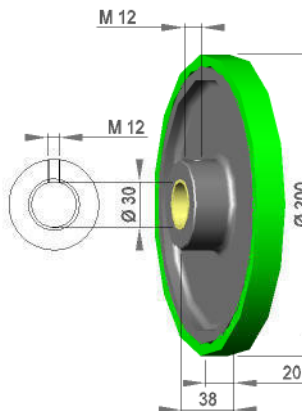
Silikon 90 shore
