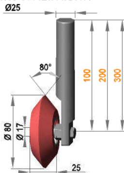
Rollenhalterung Ø25 mit Rolle ER 17 / 25 / 80 / PO
