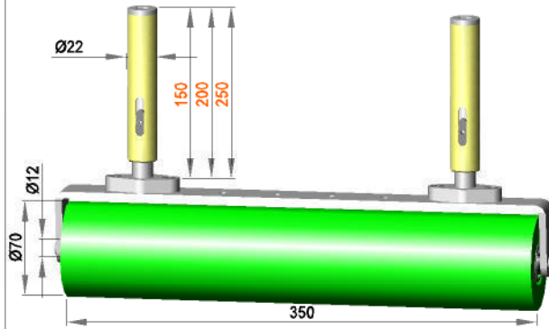
Gefederte Rollenhalterung mit Rolle R 12 / 350 / 70 / PO
