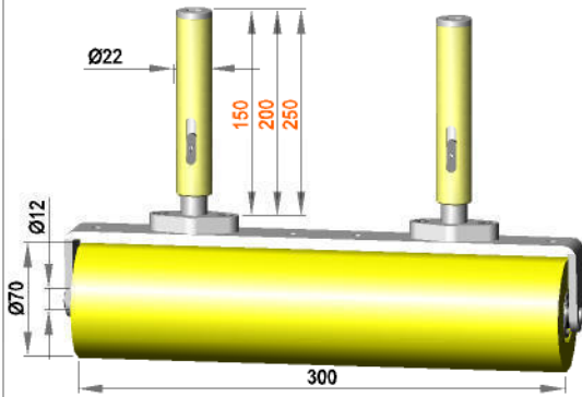
Gefederte Rollenhalterung mit Rolle R 12 / 300 / 70 / AL
