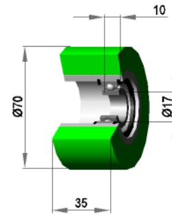
Silikon 90 shore
