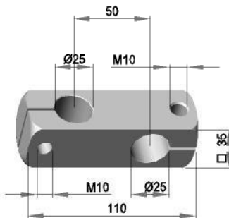
Kreuzklemmstück - rechts KRR 25 /R
