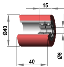
Silikon 50 shore
