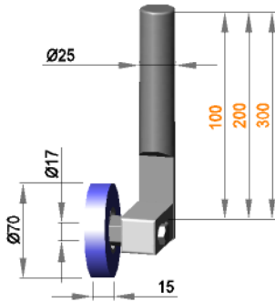
Rollenhalterung Ø25 drehbar mit Rolle R 17 / 15 / 70 / AL
