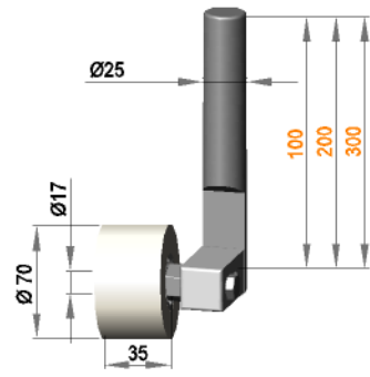
Rollenhalterung Ø25 drehbar mit Rolle R 17 / 50 / 70 / S50R
