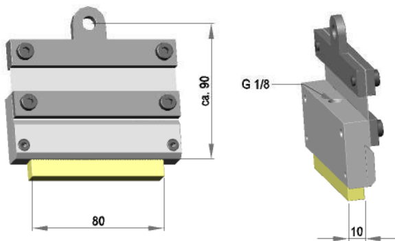
Filzhalter, Montage oben, Filz 20 mm FH / S / 20
