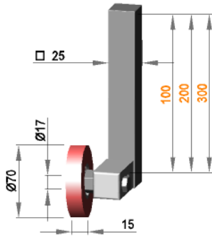
Rollenhalterung □ 25 drehbar mit Rolle R 17 / 17 / 70 / PO
