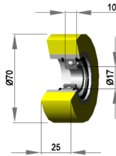
Silikon 70 shore
