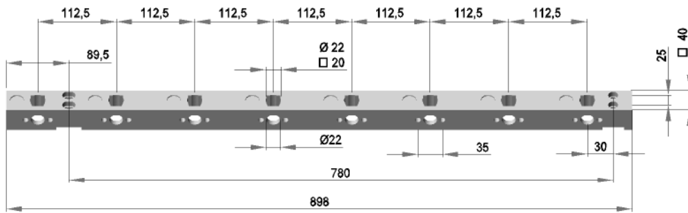
Werkzeugträger 900mm lang, Abstand 112,5 mm, rechte Ausführung
