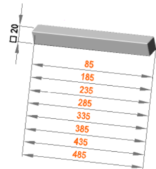
Klemmstück KG 22 / M12
