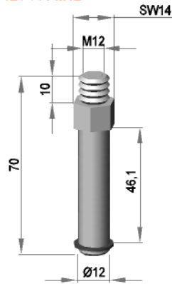
Rollenaufnahme RA 12 / 50 / M12
