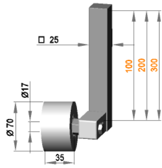
Rollenhalterung □ 25 drehbar mit Rolle R 17 / 50 / 70 / S30B
