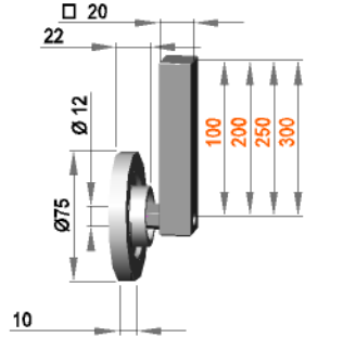
drehbare Führungsrollenhalterung mit Rolle F 12 / 10 / 75 / AL
