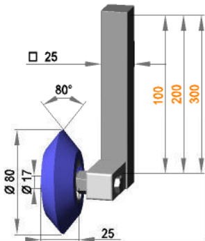
Rollenhalterung □ 25 drehbar mit Rolle ER 17 / 25 / 80 / AL
