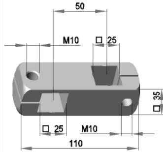
Kreuzklemmstück - links
