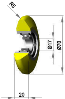
Silikon 70 shore
