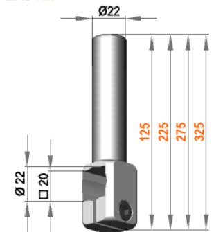
Einfachklemmstück EKU 125 EKU 225 EKU 275 EKU 325
