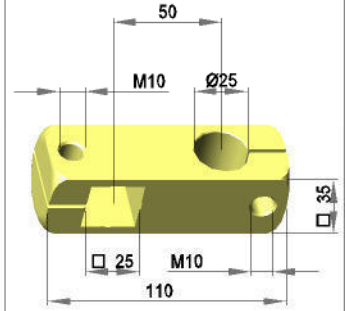
Kreuzklemmstück - links
