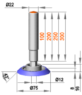
Feststehende Rollenhalterung mit Rolle ERL 12 / 16 / 45 / S30B
