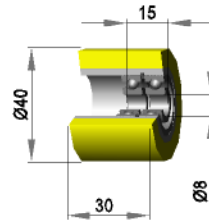
Silikon 70 shore
