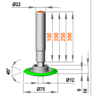
Feststehende Rollenhalterung mit Rolle ERL 12 / 18 / 80 / S90Gr
