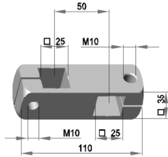
Kreuzklemmstück - rechts
