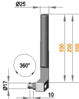
Rollenhalterung □ 25 drehbar
