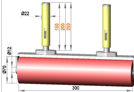
Gefederte Rollenhalterung mit Rolle R 12 / 300 / 70 / S90Gr
