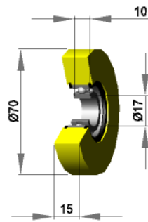
Silikon 70 shore
