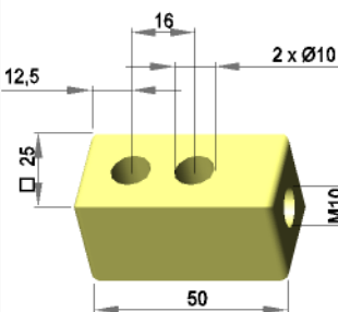
Rollenhalter
