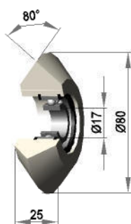
Polyamid
