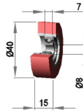
Silikon 50 shore
