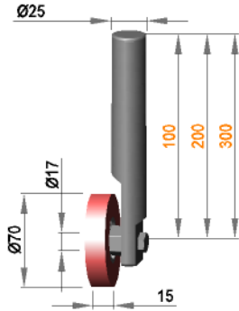
Rollenhalterung Ø25 mit Rolle R 17 / 17 / 70 / PO
