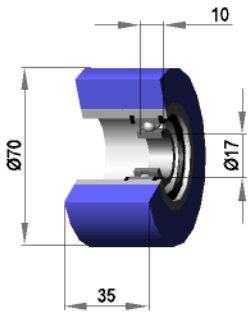
Silikon 30 shore
