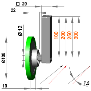
Führungsrollenhalterung □ 20 mit Rolle F 12 / 10 / 100 / S90Gr
