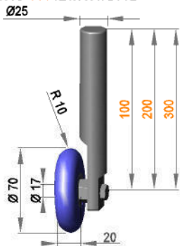
Rollenhalterung Ø25 mit Rolle RR17 / 20 / R10 / AL
