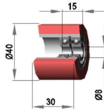
Silikon 50 shore
