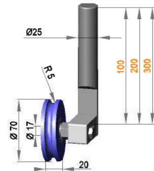
Rollenhalterung Ø25 drehbar mit Rolle NR17 / 20 / R5 / AL
