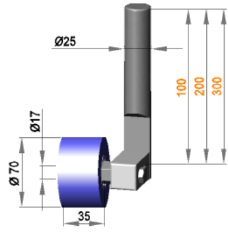
Rollenhalterung Ø25 drehbar mit Rolle R 17 / 35 / 70 / AL
