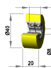
Silikon 70 shore
