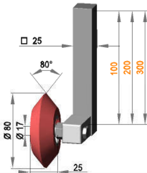
Rollenhalterung □ 25 drehbar mit Rolle ER 17 / 25 / 80 / PO
