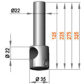
Einfachklemmstück EK 125 EK 225 EK 275 EK 325
