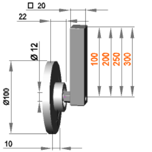
drehbare Führungsrollenhalterung mit Rolle F 12 / 10 / 100 / AL
