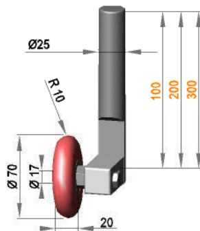
Rollenhalterung Ø25 drehbar mit Rolle RR17 / 20 / R10 / PO
