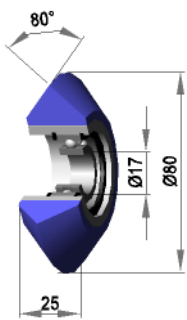
Silikon 30 shore
