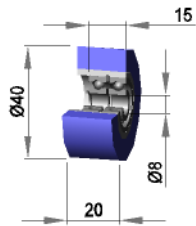
Silikon 30 shore
