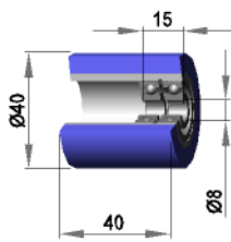
Silikon 30 shore
