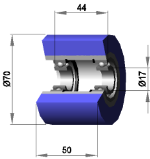
Silikon 30 shore
