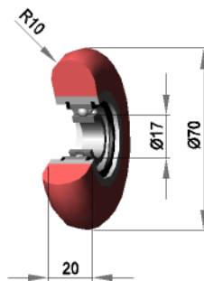
Silikon 50 shore
