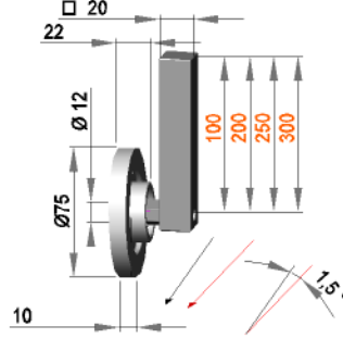
Führungsrollenhalterung 1,5° R mit Rolle F 12 / 10 / 75 / AL
