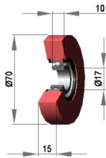
Silikon 50 shore
