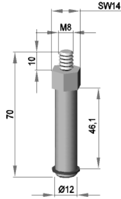
Rollenaufnahme RA 12 / 50 / M8
