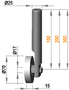
Rollenhalterung Ø25 mit Rolle R 17 / 25 / 70 / S30B
