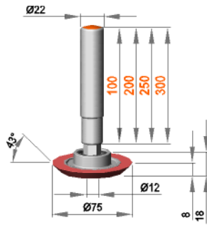
Feststehende Rollenhalterung mit Rolle ERL 12 / 16 / R43 / S50R
