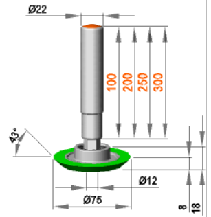
Feststehende Rollenhalterung mit Rolle ERL 12 / 16 / R43 / S90Gr
