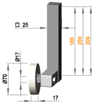
Rollenhalterung □ 25 drehbar mit Rolle R 17 / 25 / 70 / S50R
