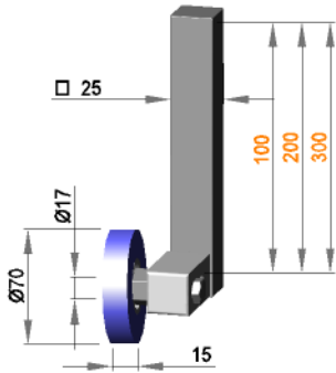
Rollenhalterung □ 25 drehbar mit Rolle R 17 / 15 / 70 / AL
