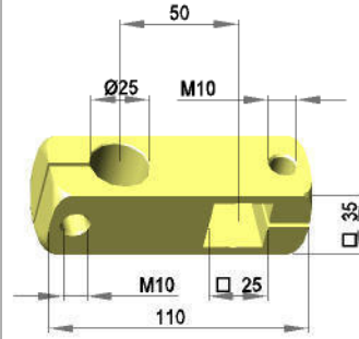
Kreuzklemmstück - rechts
