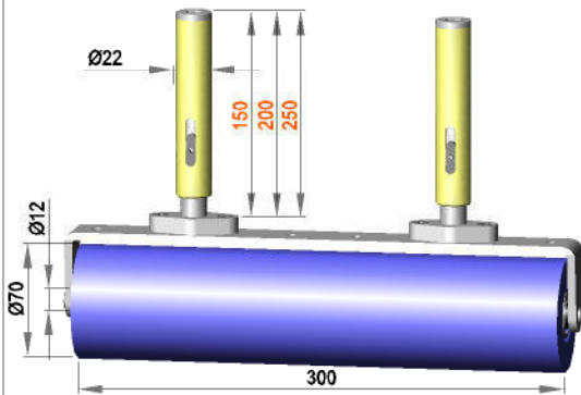
Gefederte Rollenhalterung mit Rolle R 12 / 300 / 70 / S70G
