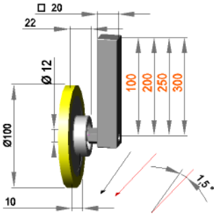
Führungsrollenhalterung 1,5° R mit Rolle F 12 / 10 / 100 / S70G
