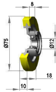
Silikon 70 shore
