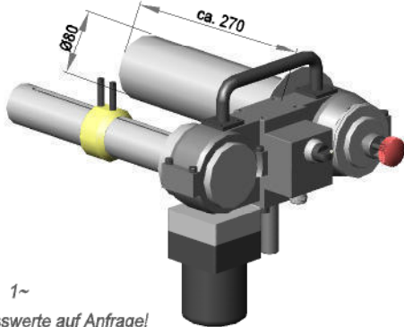
Restfolienwickler, zum Abziehen und Aufwickeln der abgeschnittenen Dekormaterialien, linke Ausführung
