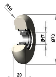
Polyamid
