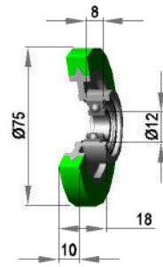
Silikon 90 shore
