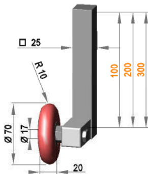
Rollenhalterung □ 25 drehbar mit Rolle RR17 / 20 / R10 / PO
