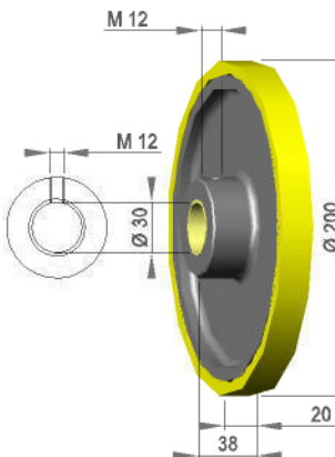
Silikon 70 shore
