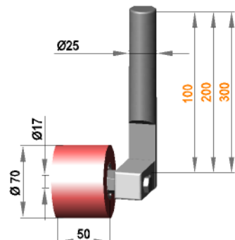
Rollenhalterung Ø25 drehbar mit Rolle R 17 / 50 / 70 / PO
