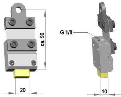
gefederter Filzhalter, Montage oben, Filz 80 mm FH / G / 80
