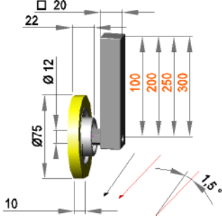
Führungsrollenhalterung 1,5° R mit Rolle F 12 / 10 / 75 / S70G
