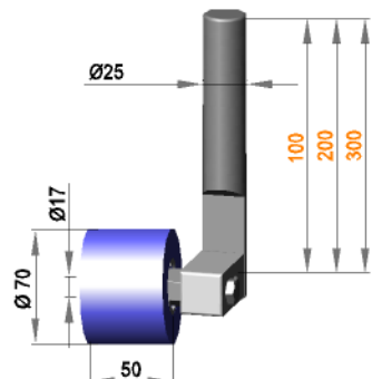
Rollenhalterung Ø25 drehbar mit Rolle R 17 / 50 / 70 / AL
