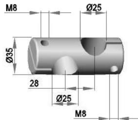
Kreuzklemmstück - rechts RRR 25 /R
