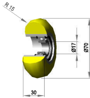
Silikon 70 shore
