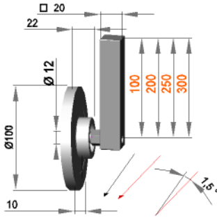
Führungsrollenhalterung 1,5° R mit Rolle F 12 / 10 / 100 / AL
