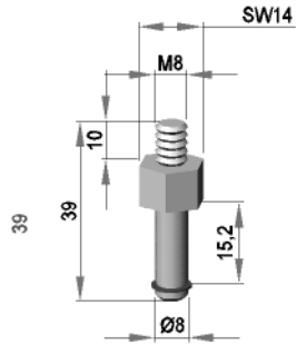
Rollenaufnahme RA 8 / 20 / M8
