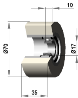
Polyamid
