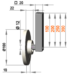
drehbare Führungsrollenhalterung mit Rolle F 12 / 10 / 100 / PO
