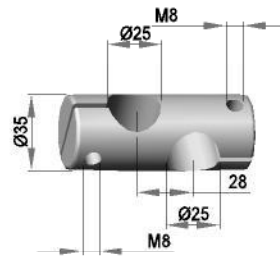
Kreuzklemmstück - links RRR 25 /L
