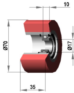
Silikon 50 shore
