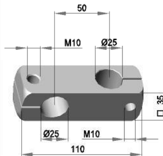
Kreuzklemmstück - links KRR 25 /L
