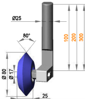
Rollenhalterung Ø25 drehbar mit Rolle ER 17 / 25 / 80 / AL
