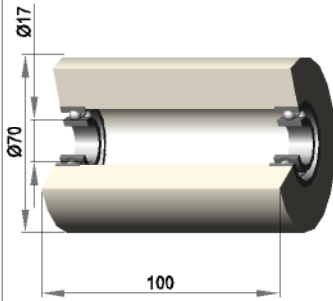
Polyamid
