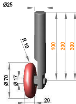
Rollenhalterung Ø25 mit Rolle RR17 / 20 / R10 / PO
