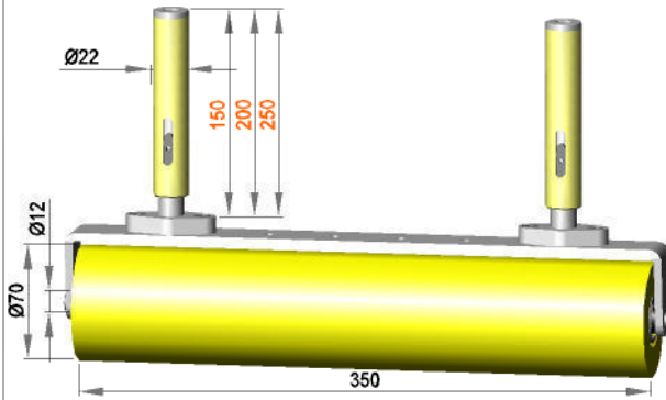
Gefederte Rollenhalterung mit Rolle R 12 / 350 / 70 / AL
