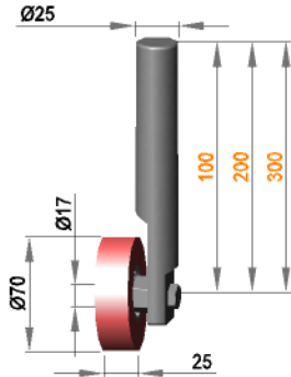
Rollenhalterung Ø25 mit Rolle R 17 / 25 / 70 / PO
