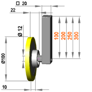
drehbare Führungsrollenhalterung mit Rolle F 12 / 10 / 100 / S70G
