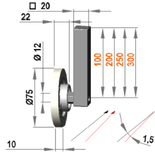
Führungsrollenhalterung □ 20 mit Rolle F 12 / 10 / 75 / PO
