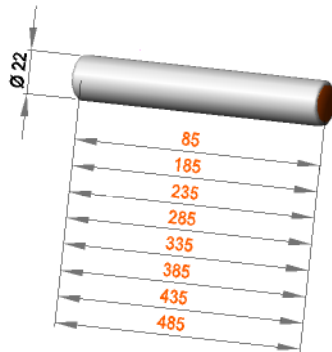
Befestigungsstück KF 22 / 80 / M8
