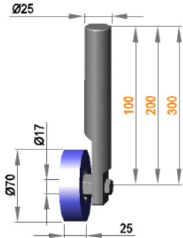
Rollenhalterung Ø25 mit Rolle R 17 / 25 / 70 / AL
