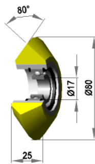
Silikon 70 shore
