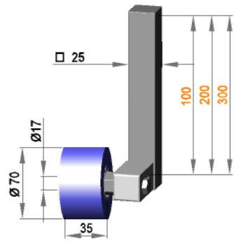
Rollenhalterung □ 25 drehbar mit Rolle R 17 / 35 / 70 / AL
