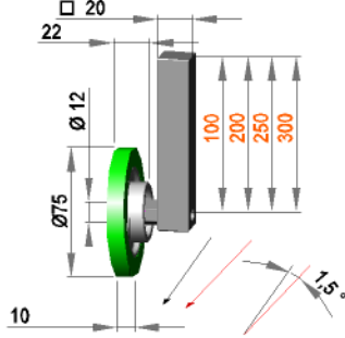
Führungsrollenhalterung 1,5° R mit Rolle F 12 / 10 / 75 / S90Gr
