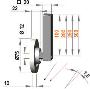
Führungsrollenhalterung 1,5° R mit Rolle F 12 / 10 / 75 / PO
