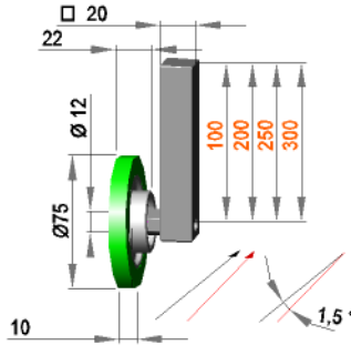
Führungsrollenhalterung □ 20 mit Rolle F 12 / 10 / 75 / S90Gr
