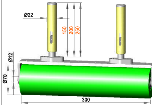
Gefederte Rollenhalterung mit Rolle R 12 / 300 / 70 / PO
