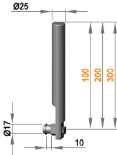
Rollenhalterung □ 25
