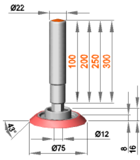
Feststehende Rollenhalterung mit Rolle ERL 12 / 16 / 45 / S50R
