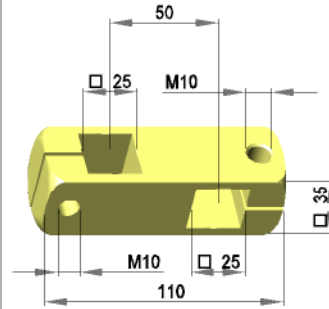
Kreuzklemmstück - rechts
