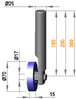
Rollenhalterung Ø25 mit Rolle R 17 / 15 / 70 / AL
