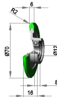
Silikon 90 shore
