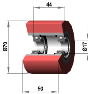
Silikon 50 shore
