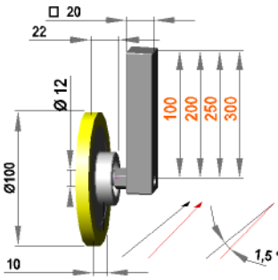
Führungsrollenhalterung □ 20 mit Rolle F 12 / 10 / 100 / S70G
