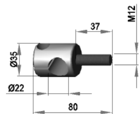
Klemmstück KG 22 / M12
