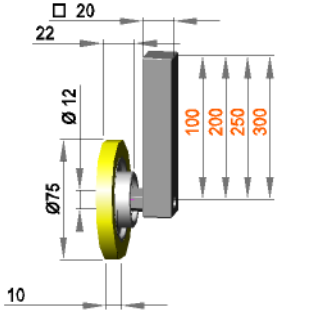
drehbare Führungsrollenhalterung mit Rolle F 12 / 10 / 75 / S70G
