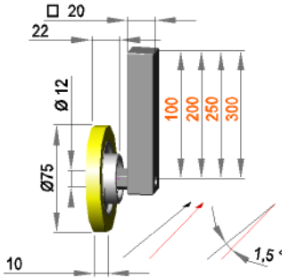
Führungsrollenhalterung □ 20 mit Rolle F 12 / 10 / 75 / S70G
