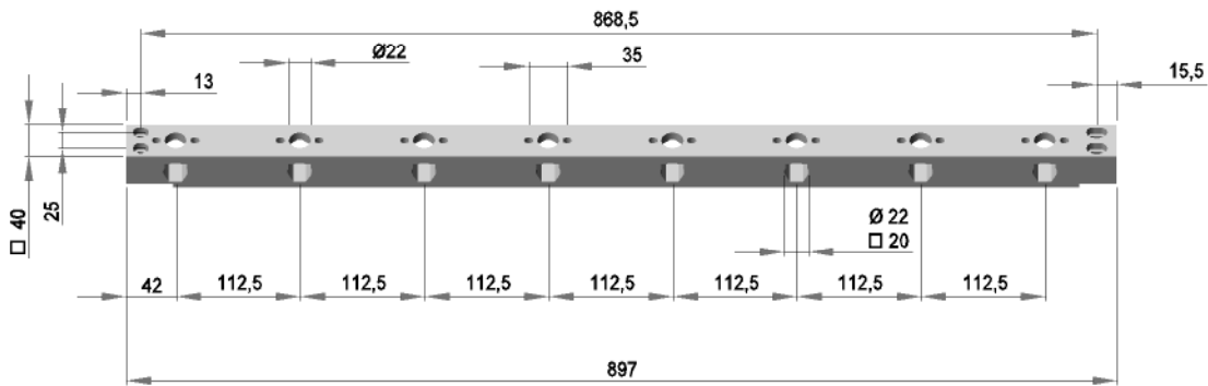
Werkzeugträger für Höhenverstellung
