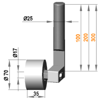
Rollenhalterung Ø25 drehbar mit Rolle R 17 / 50 / 70 / S30B
