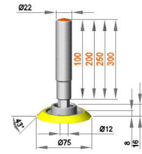
Feststehende Rollenhalterung mit Rolle ERL 12 / 16 / 45 / S70G
