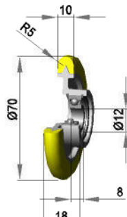
Silikon 70 shore
