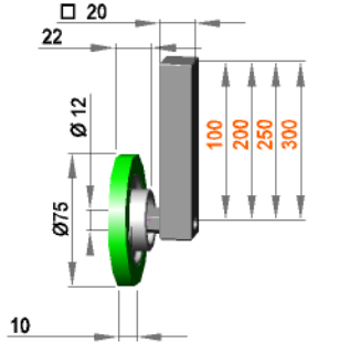
drehbare Führungsrollenhalterung mit Rolle F 12 / 10 / 75 / S90Gr
