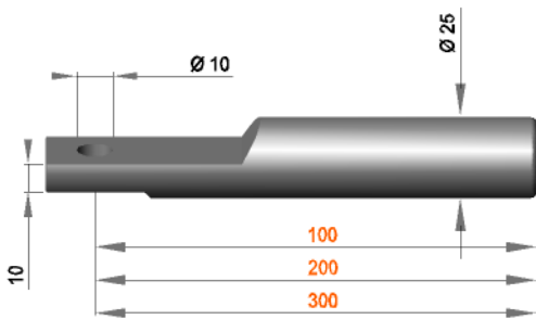
Rollenhalter
