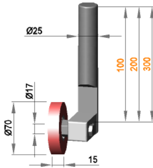
Rollenhalterung Ø25 drehbar mit Rolle R 17 / 17 / 70 / PO
