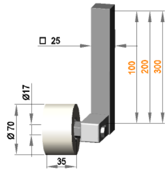
Rollenhalterung □ 25 drehbar mit Rolle R 17 / 50 / 70 / S50R
