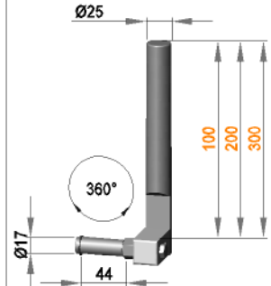
Rollenhalterung □ 25 drehbar
